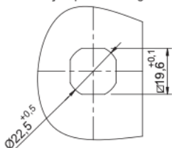
Furação para montagem
