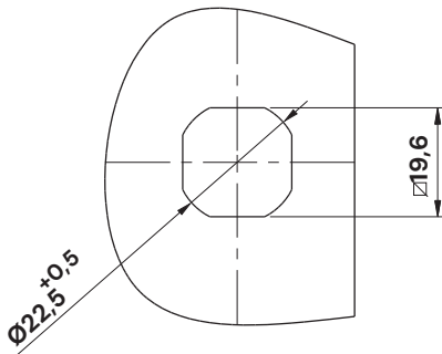
Perforación para Montaje
