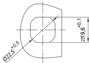
Furação para montagem
