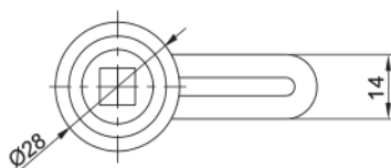
Furação para montagem
