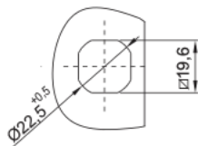
Furação para montagem
