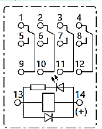
4C con indicador y diodo
